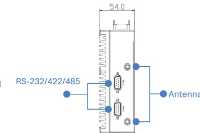
Top I/O
